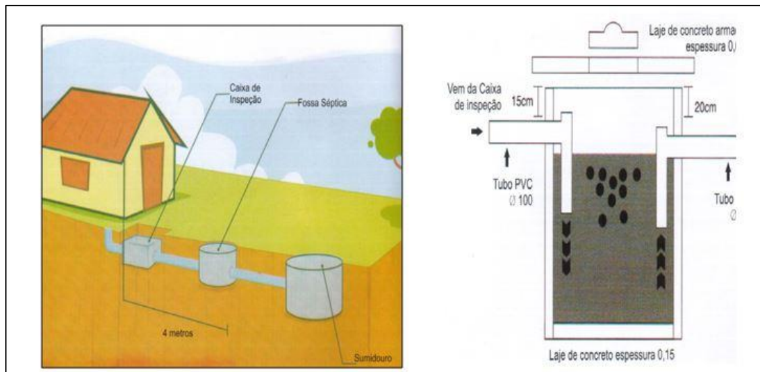
Figura 84 - Sistema Individual de Tratamento – Fossas Sépticas.
