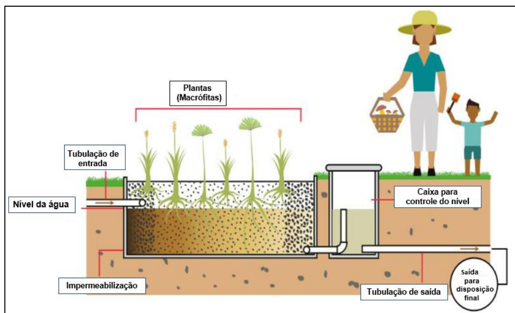
Figura 90 - Esquema de zona de raízes ou SAC.
