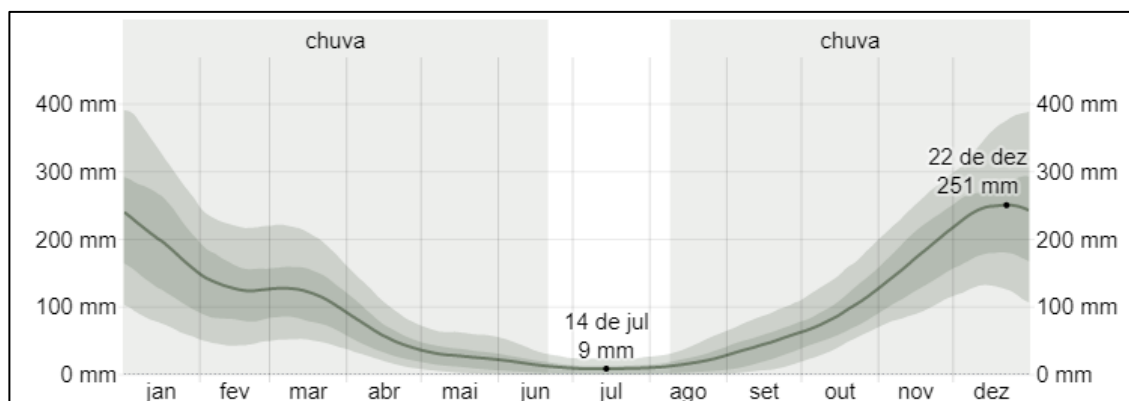
Figura 6 – Gráfico de Precipitação em Recreio.
