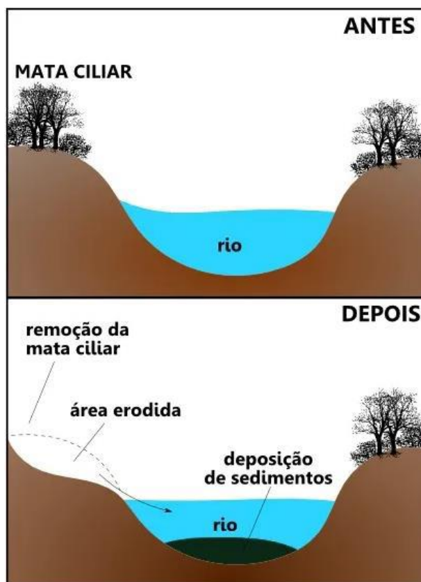
Figura 122 - Esquema de Assoreamento.
