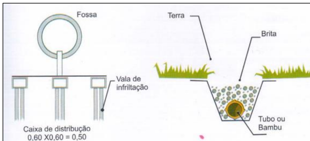
Figura 85 – Sistema de tratamento individual – Valas de Infiltração.
