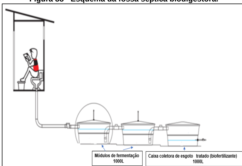
Figura 88 - Esquema da fossa séptica biodigestora.
