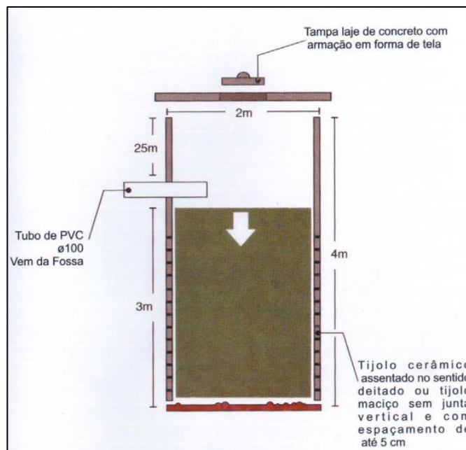
Figura 86 – Sistema individual de tratamento – Sumidouro.
