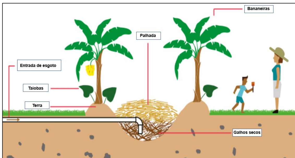
Figura 92 - Esquema de círculo de bananeira.
