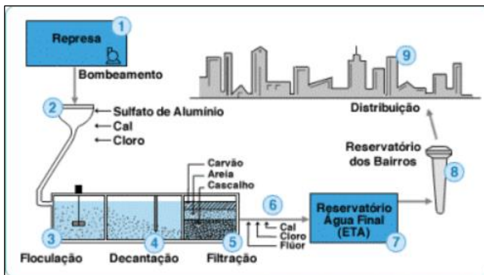
Figura 30 – Etapas de tratamento de uma ETA convencional.
